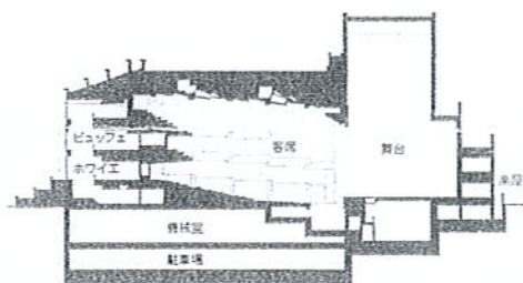
大ホール断面図
